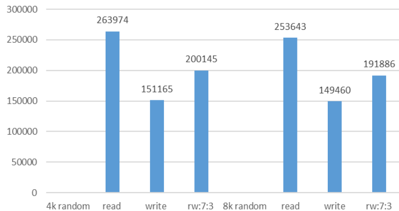
1 volume iops
