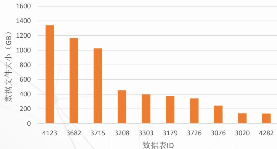
数据量Top10
