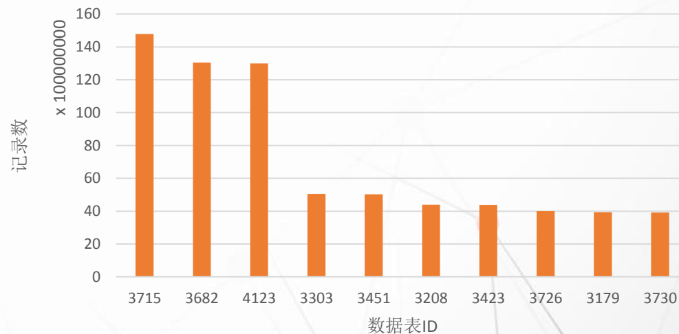
记录数Top 10
