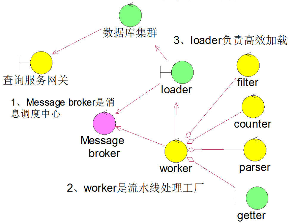
基于流处理的大数据处理框架
