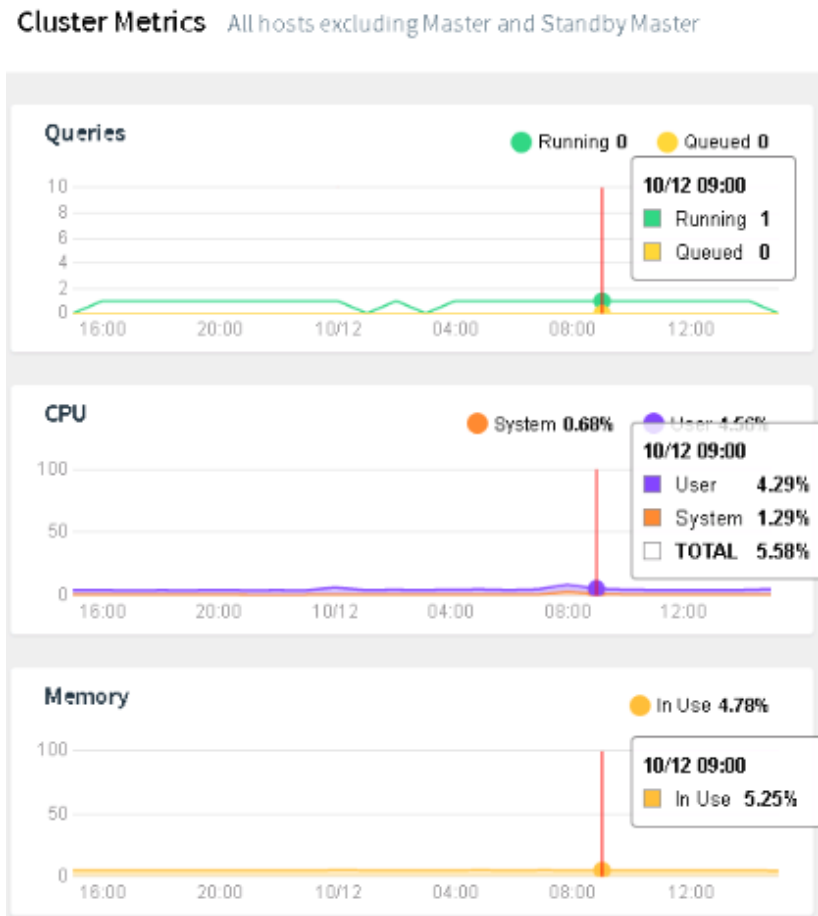
利用GCC监控
