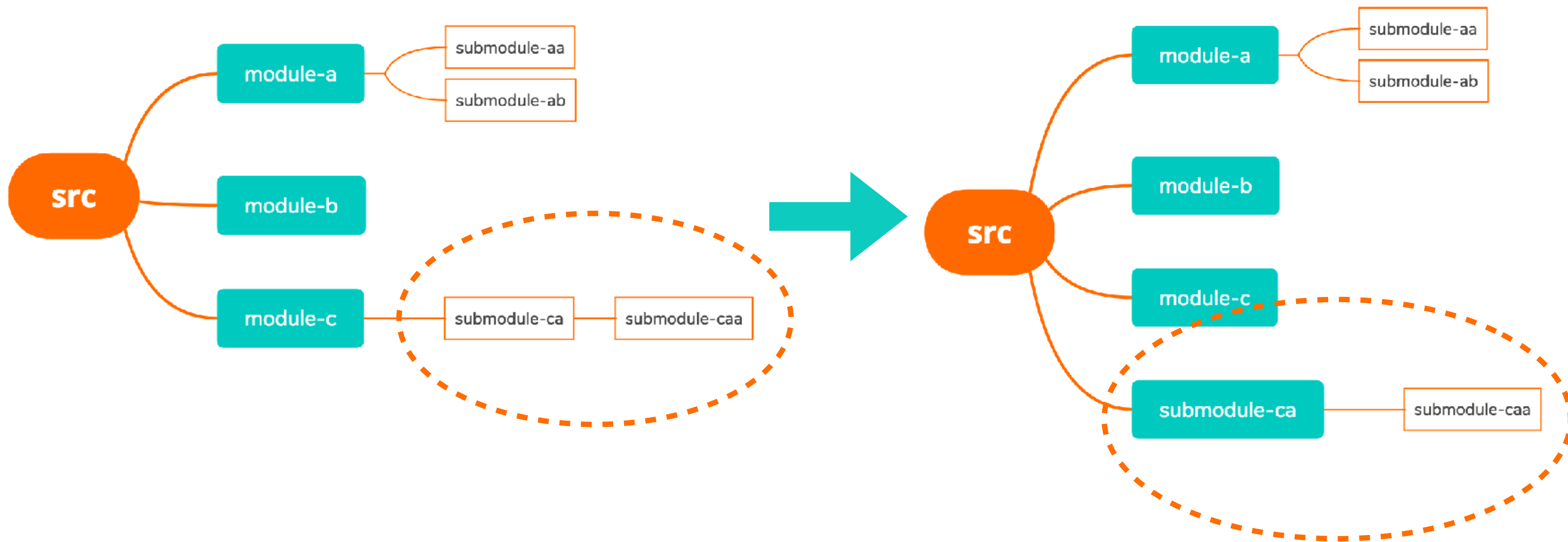
Node.js 模块关系
