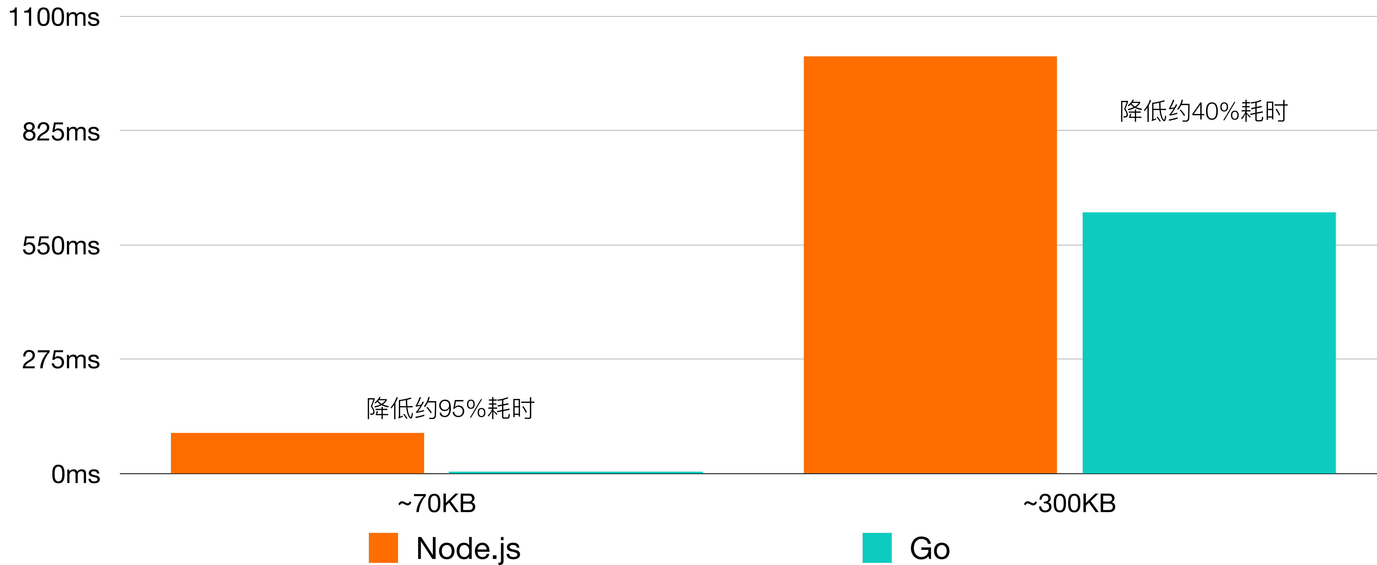
相同diff算法、文件样本下的耗时对比
